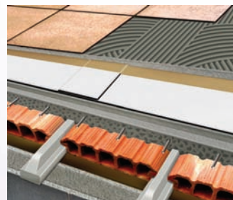
Lajes transitáveis em geral, planas ou inclinadas
